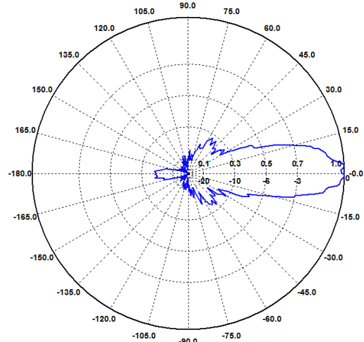
H-Ebene / H-Plane 3800 MHz
