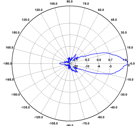
H-Ebene / H-Plane 3400 MHz
