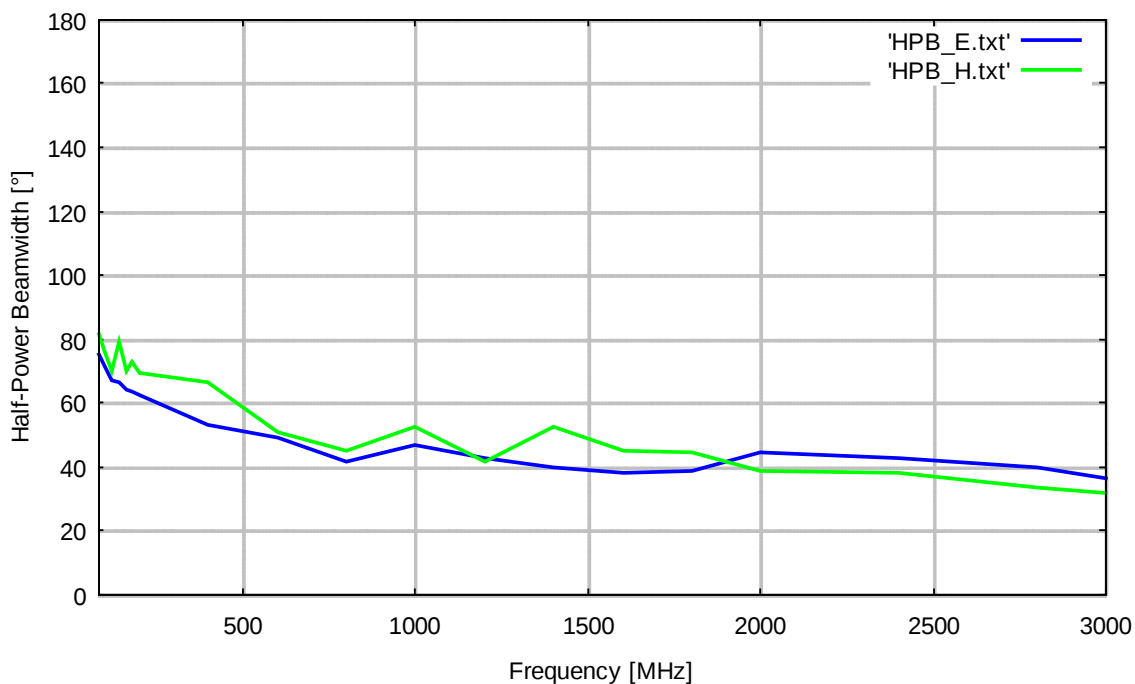
3 dB Öffnungswinkel [°]
